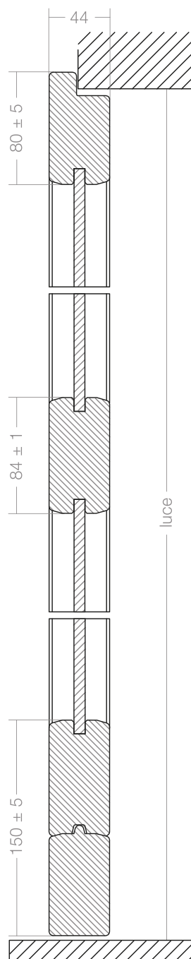
FINESTRA sezione verticale
