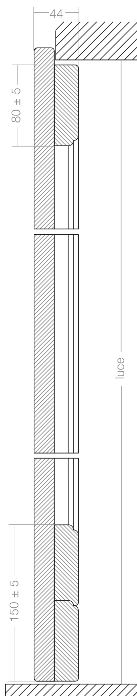
FINESTRA sezione verticale
