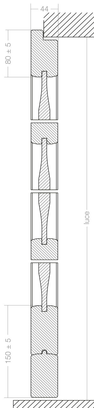
PORTA sezione verticale
