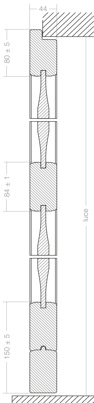
FINESTRA sezione verticale
